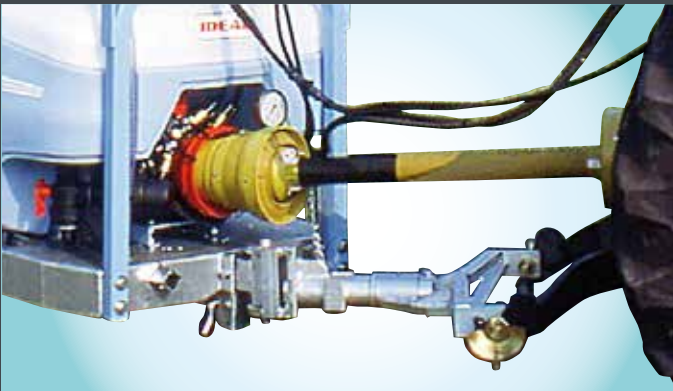
Timone articolato / Tracker drawbar / Kormányzott vonórúd / Gelenkdeichsel / Tiro articulado
