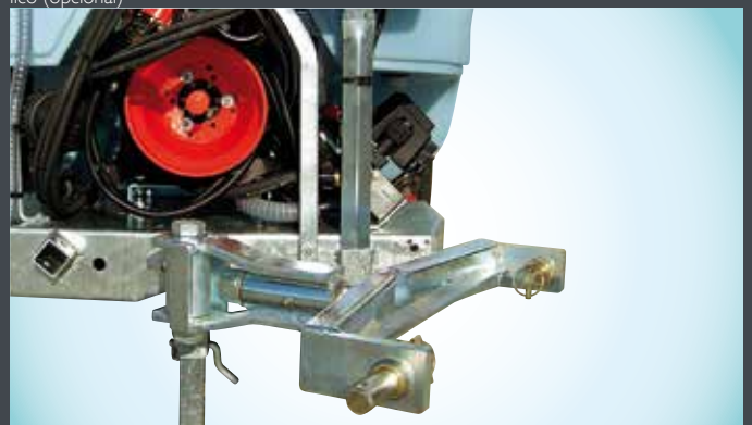
Timone articolato con cuscinetti / Tracker drawbar with bearings / Kormányzott vonórúd csapágyakkal / Gelenkdeichsel mit Lager / Tiro articulado con cojinetes
