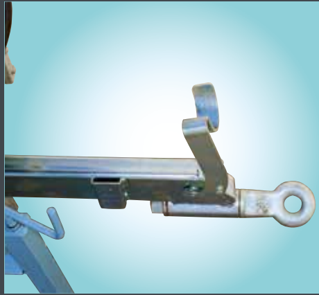
Timone a occhione / Ring drawbar / Vonószeres vonórúd Deichsel mit Öse / Tiro con gancho de arrastre
