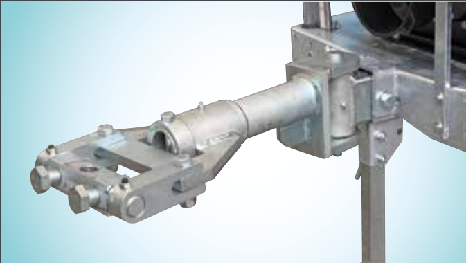
Timone sterzante con cuscinetti tipo Germania / Tracker drawbar with bearings "German type" / „Német típusú” csapágyas vonórúd / Lenkdeichsel mit Lager Germania Modell / Tiro articulado con cojinetes tipo Alemania
